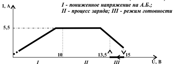
Вольт-Амперная характеристика работы НПП Орион-150 (схематично)
